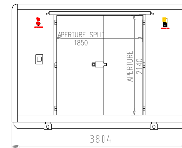
END ELEVATION
