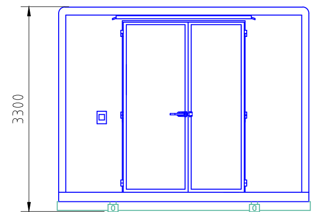
DOOR ELEVATION
